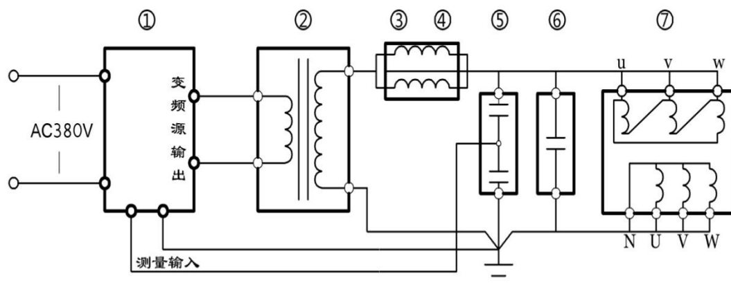
变压器耐压试验接线图
