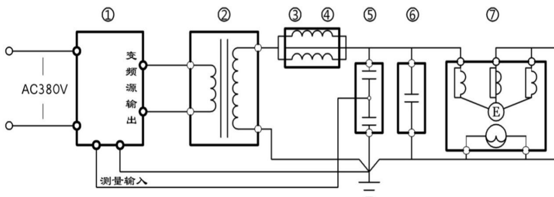
发电机耐压试验接线图
